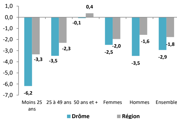
Evolution annuelle (T1 2020/T1 2019) des DEFM cat. ABC en fonction du sexe et de l'âge (en %)
